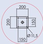
Uhr zweiseitig mit Deckenabhangung „DA“
