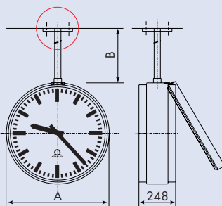
Uhr zweiseitig mit Deckenabhangung „DA“
