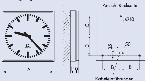
Uhr einseitig für Wandmontage „W“
