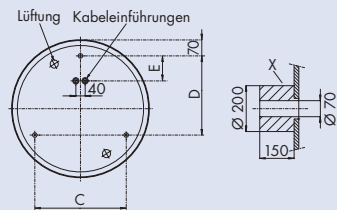
Ansicht Rückseite
