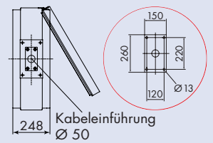
Uhr zweiseitig mit Wandarm „WA“
