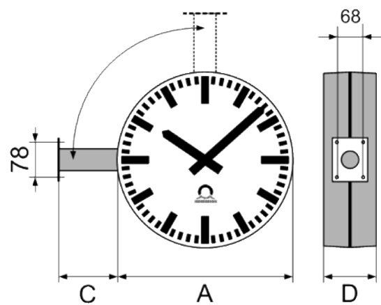
Montageset „WA“ und „DA“: (nicht für Option BW und DD)
