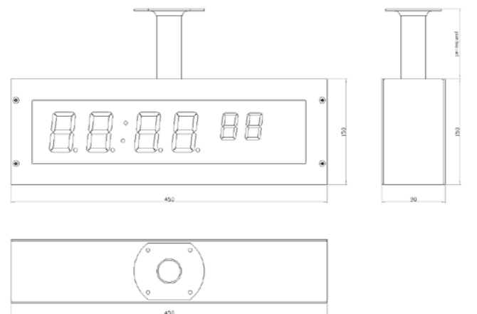
doppelseitige Ausführung
