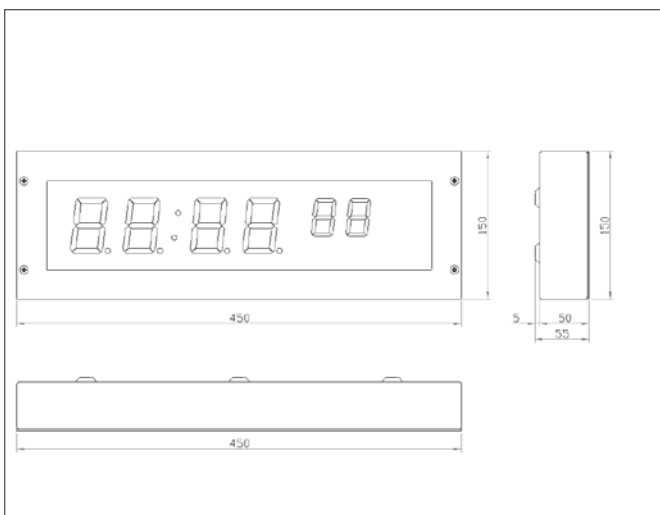
einseitige Ausführung
